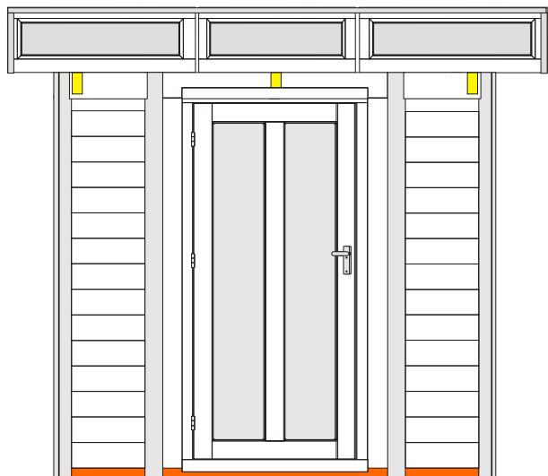
VOORAANZICHT
