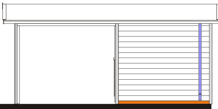
Zijaanzicht zijwand: 180-240-300-360 + voordak 310
